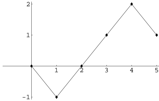
Figura 1: Una trayectoria del paseo al azar
